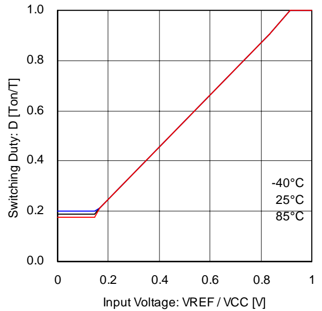
Fig.14 VREF - DUTY(VCC=12V)
